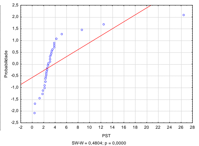
Figura 23. Gráficos Box-Plot e teste de Normalidade de Shapiro-Wilk dos atributos químicos do solo (pH, K, V, Na e PST).
