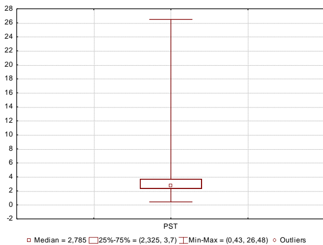
Figura 23. Gráficos Box-Plot e teste de Normalidade de Shapiro-Wilk dos atributos químicos do solo (pH, K, V, Na e PST).
