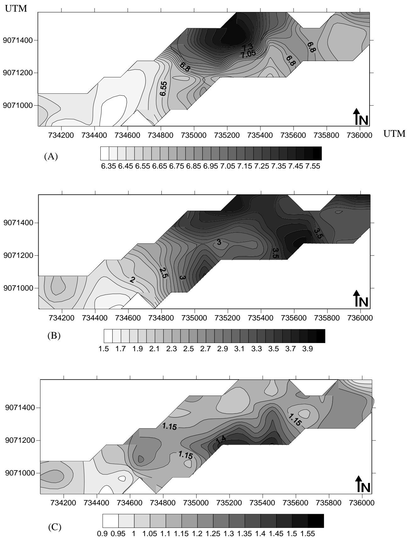
Figura 25. Mapas de isolinhas dos atributos químicos do solo: (A) pH, (B) magnésio, (C) acidez potencial.
